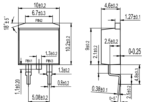
TO-263(D 2 PAK) HER10XXBCT
